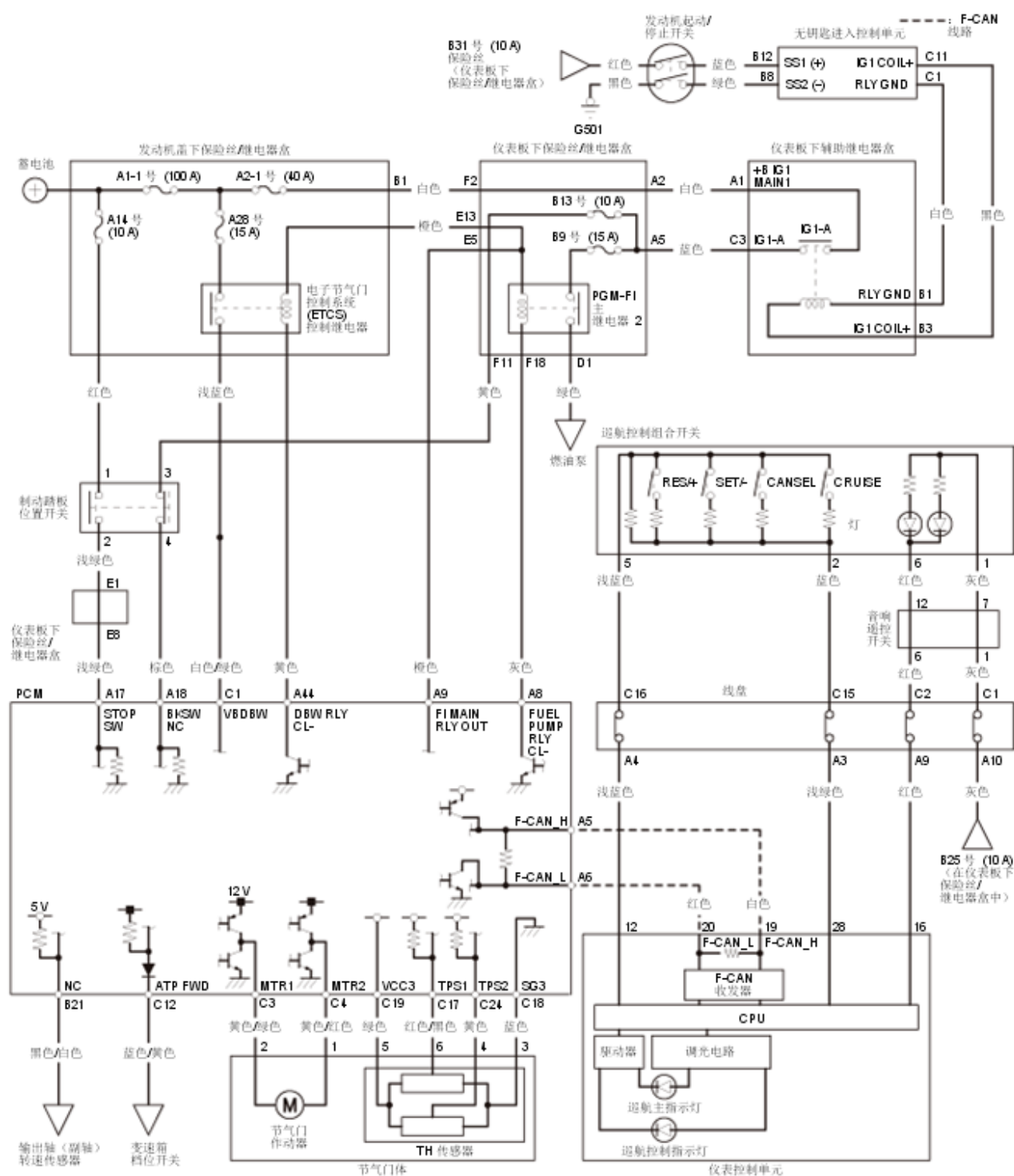
巡航控制电路图
